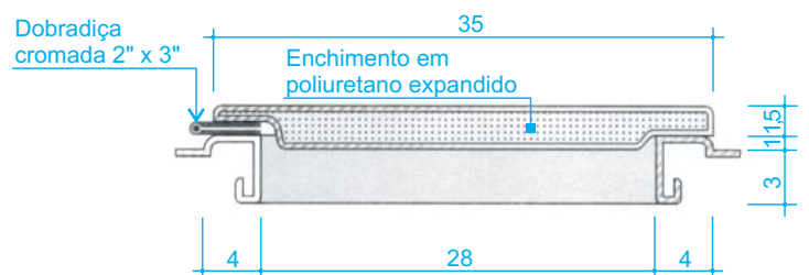
DETALHE DA TAMPA DA ÁREA DE GELADOS
