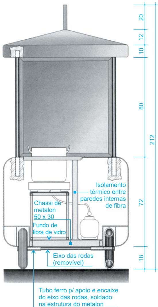
CORTE BB
