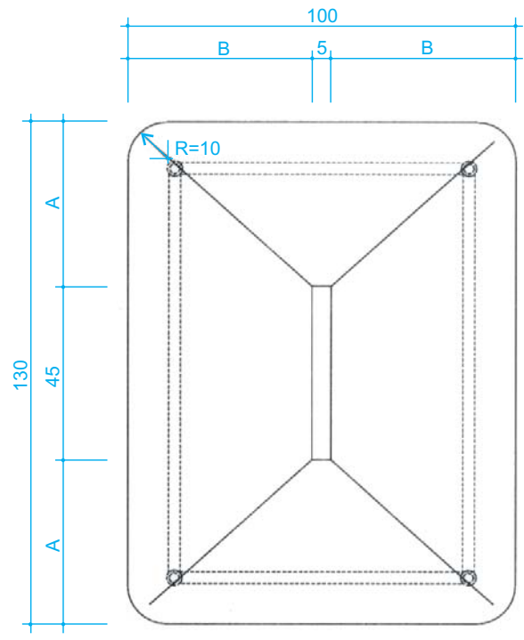
COBERTURA
