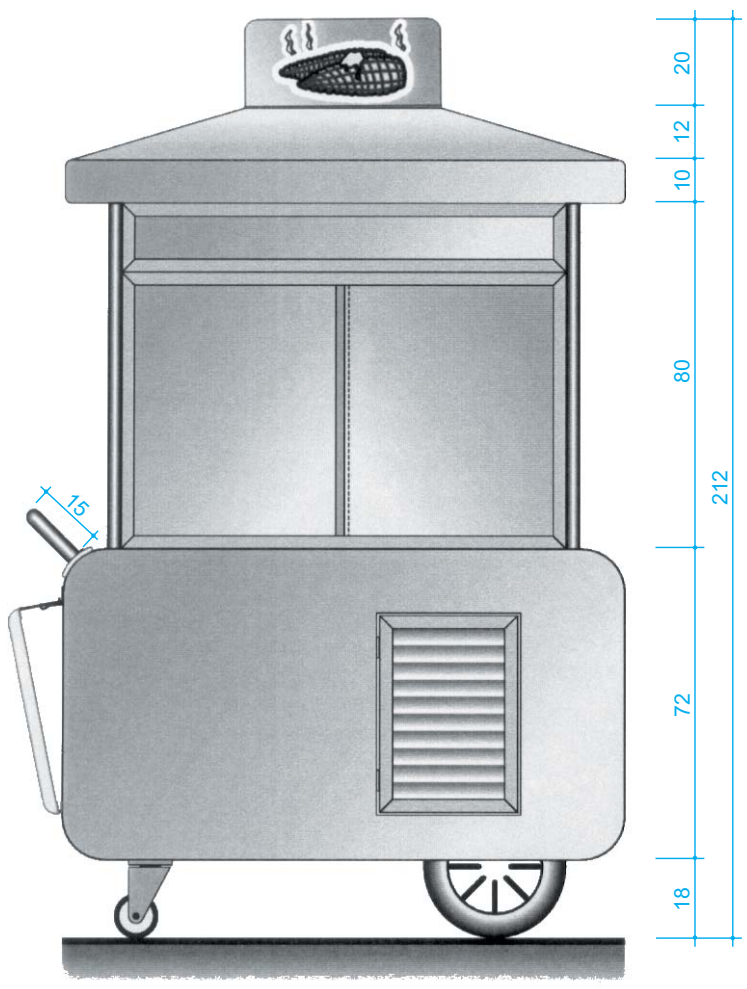
VISTA LATERAL
